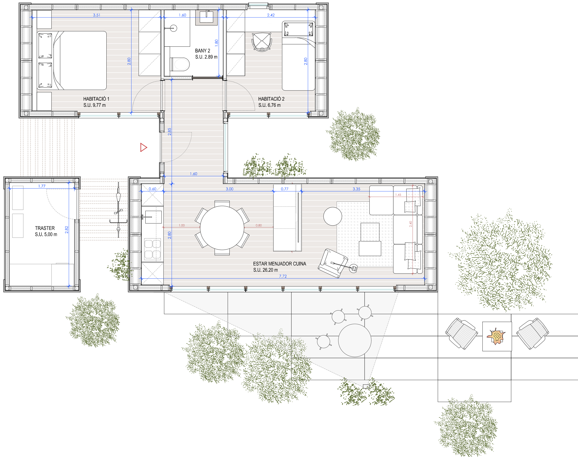
PLANTA BAIXA (E:1/50)
